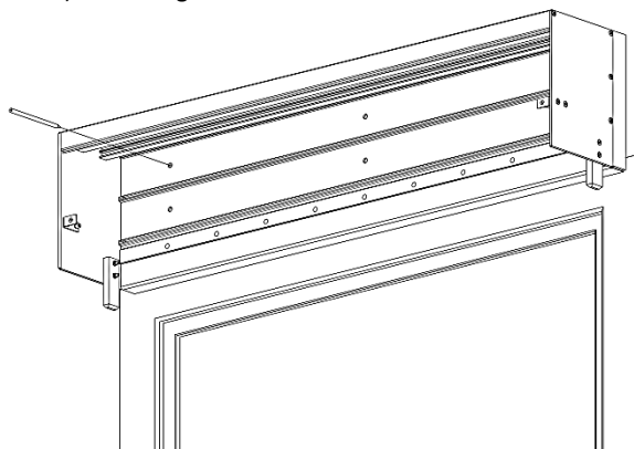
Zeichn. 14. Schema zur Ausführung der Bohrlöcher in der Führungsschiene
