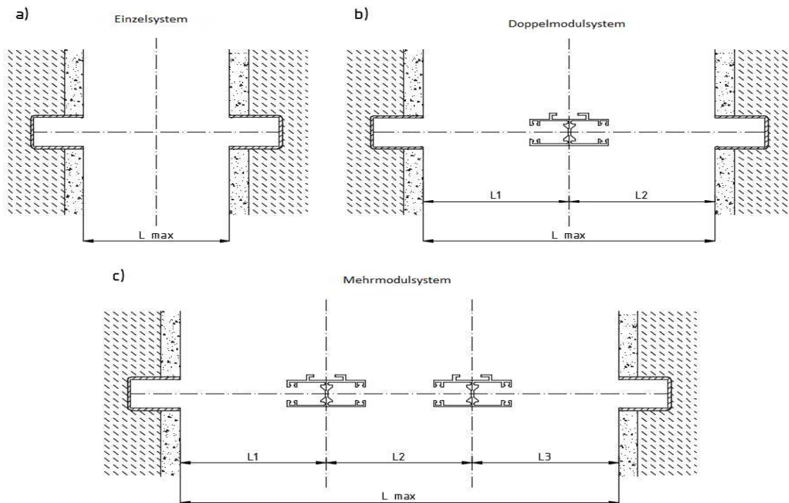
Zeichn. 4 Aufmaß: a) - Einzelsystem, b) - Doppelmodulsystem, c) Mehrmodulsystem.
