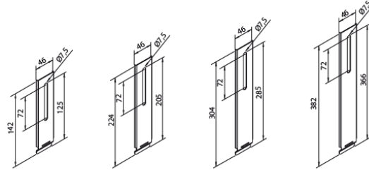
Blendenhilfshalter (4 Größen)
