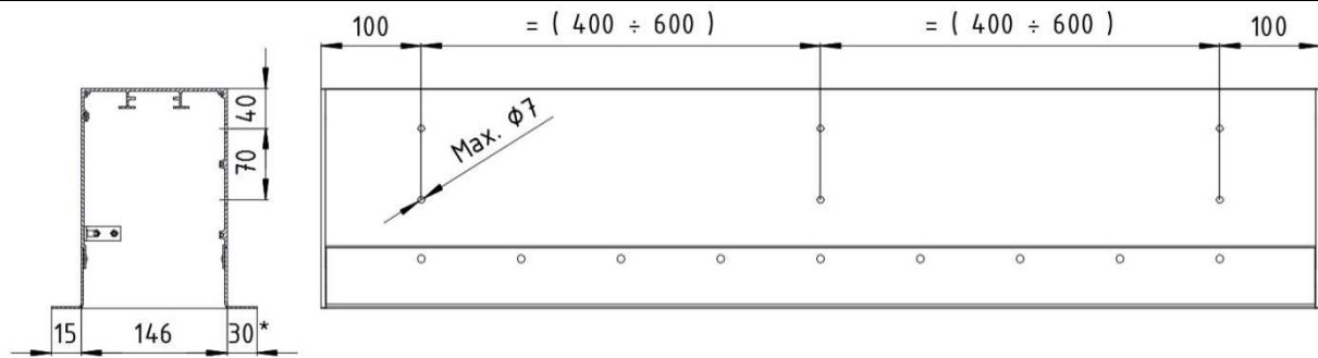
Zeichn. 13. Schema zur Ausführung der Bohrlöcher in der Unterputzkassette * - 30mm bei Box 2 und 4
