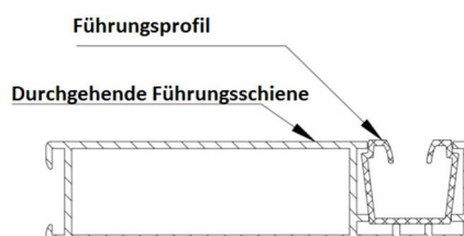
Zeichn. 5. Durchgehende Führungsschiene - Elemente
