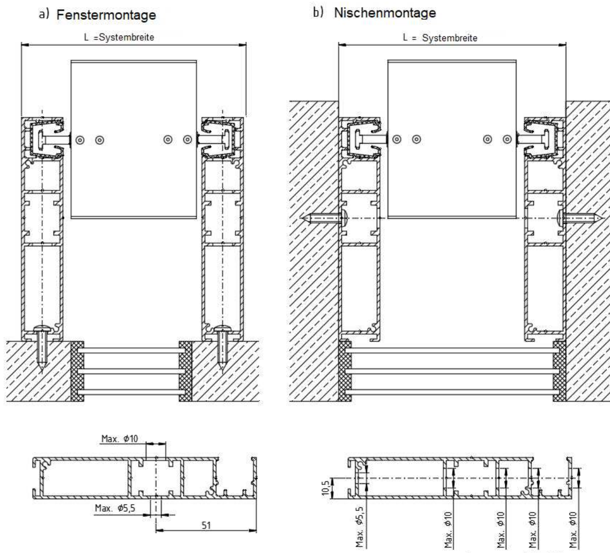
Zeichn. 12. Montageart der durchgehenden Führungsschiene: a) – Fenstermontage b) – Nischenmontage
