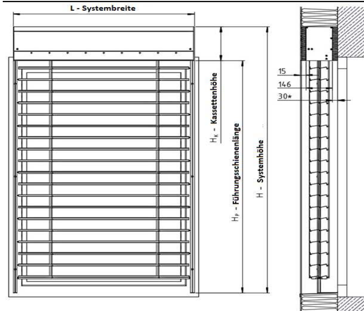
Zeichn. 11. Systemabmessungen der Raffstoren Z90 BOX - Unterputz. * - 30mm bei Box 2 und 4
