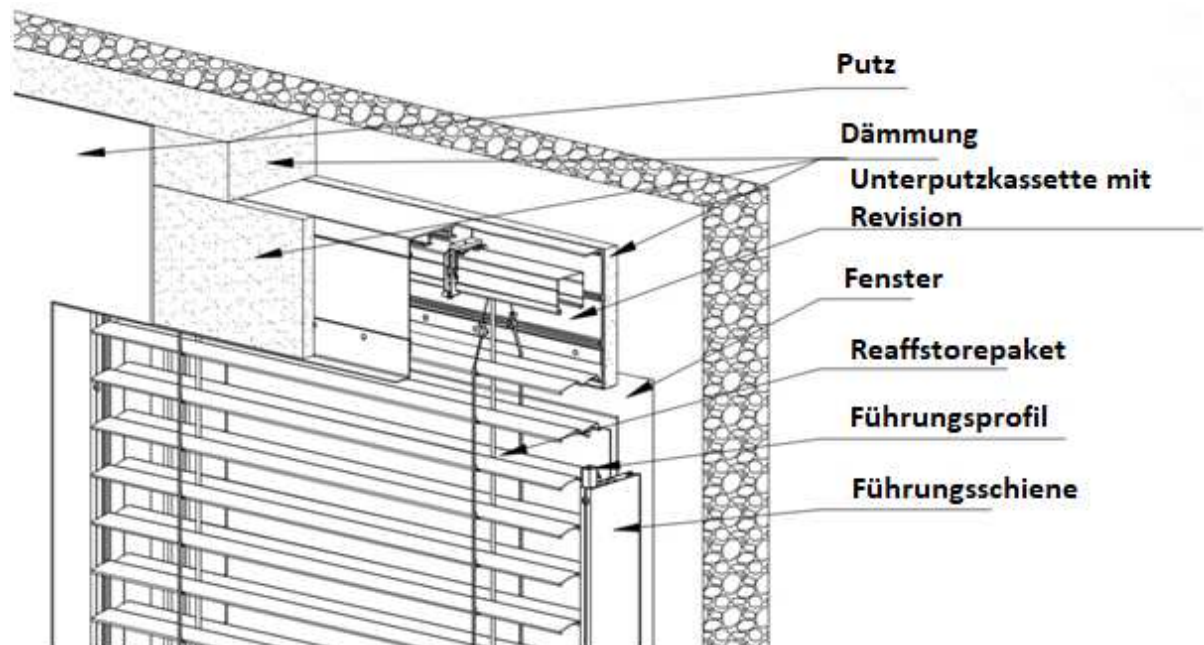
Zeichn. 10. Veranschaulichung des Raffstorensystems Z90 BOX Unterputz.
