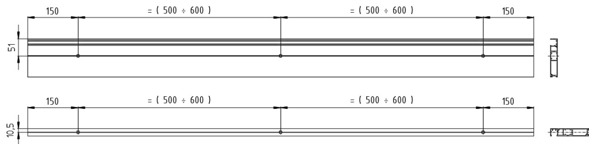
Zeichn. 14. Schema zur Ausführung der Bohrlöcher in der Führungsschiene
