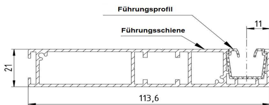
Zeichn. 9. Führungsschiene für das BOX 2 System
